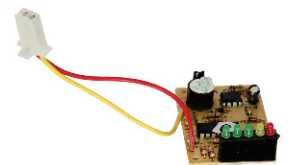
Kontrol Sirkuit + Meteran Indikasi Kapasitas Baterai
